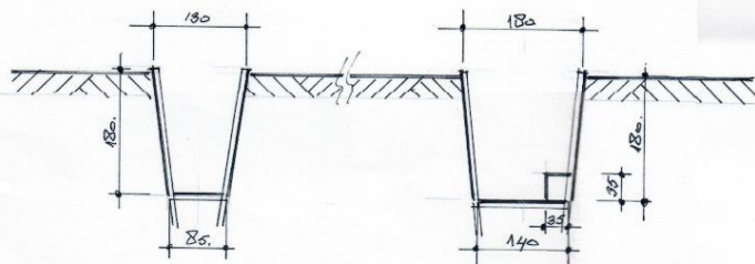
- doorsnede A -
